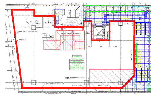
▲平面図 (1F)
