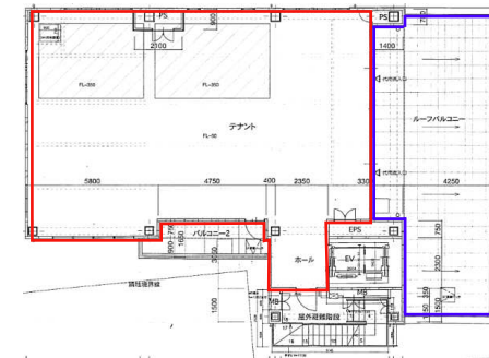
▲6F 平面図
