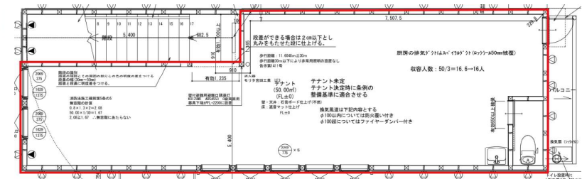
▲2F 平面図
